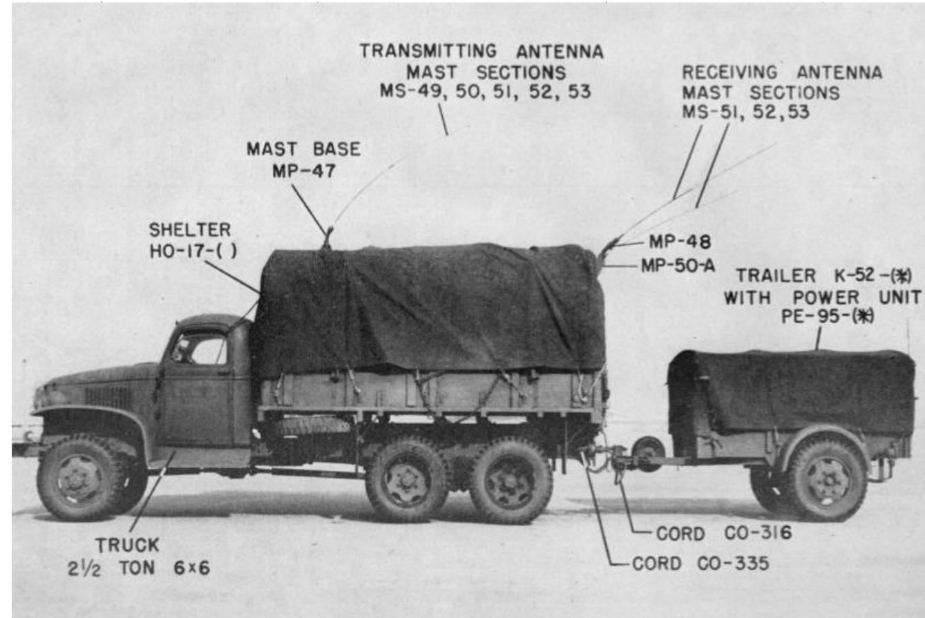
רק"ש עוצמה גבוהה 400 ואט SCR-399
