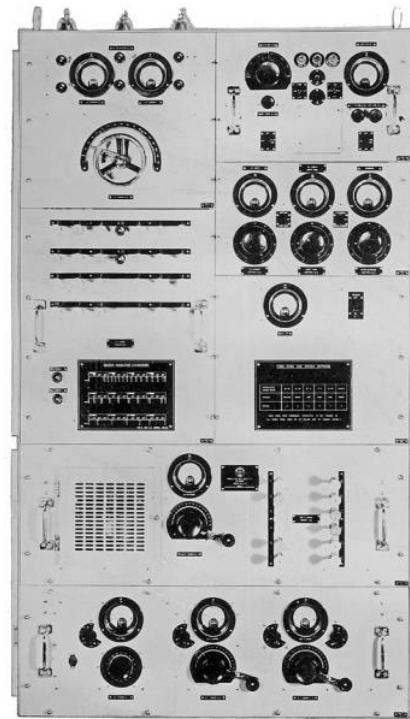
משדר 500 ואט Wireless Set No.5
