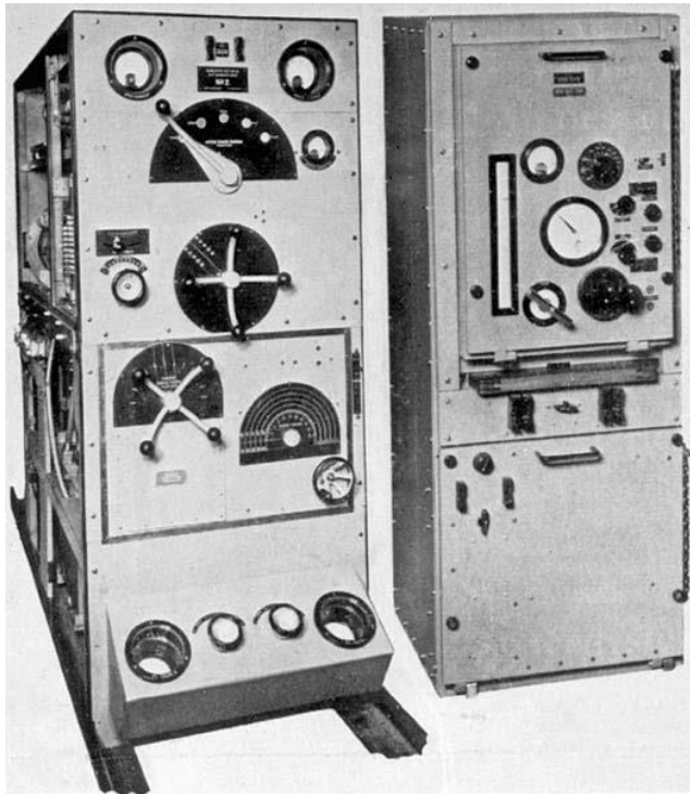
משדר 1,500 ואט Wireless Set No.16
